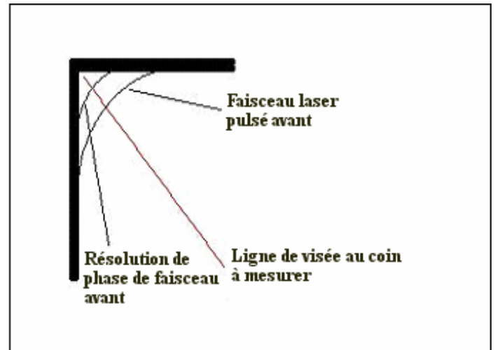
Figure 6: Effet de mesure des coins DR
