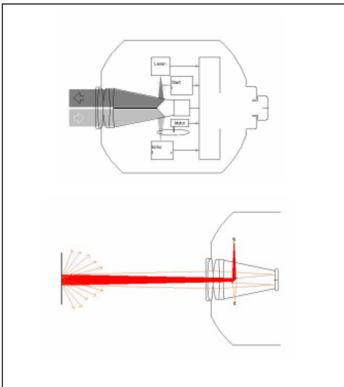
Figure 1: Principes optiques de la mesure (EDM) par laser pulsé (haut) et par déphasage (bas).
