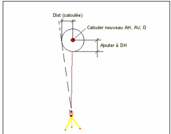
Figure 8: Mesure d'un point excentré
