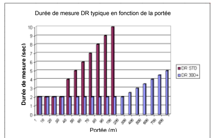
Figure 5: Durée de mesure en fonction de la portée
